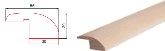
Listwa zakończeniowa
