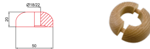
Listwa dylatacyjna
