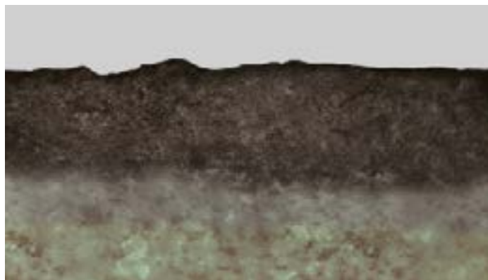
Przekrój Nadury, element silnie wzmocnionej warstwy ścieralnej połączonej ze specjalną płytą, widok spod mikroskopu elektronowego.
