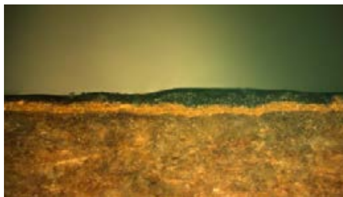
Przekrój wierzchniej warstwy podłogi laminowanej składający się z warstwy kryjącej, papieru dekoracyjnego i warstwy HDF, widok spod mikroskopu elektronowego.
